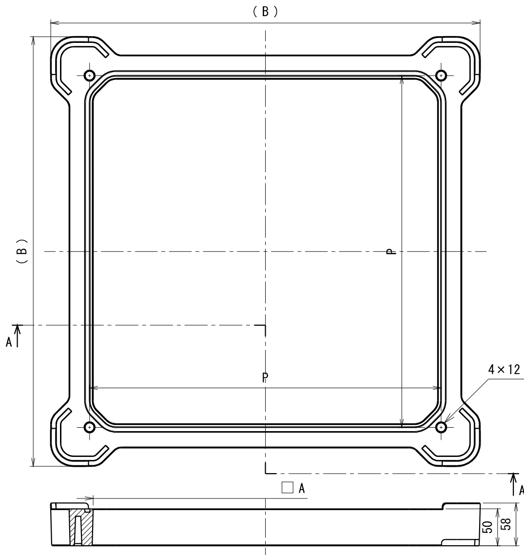
断面 A-A
