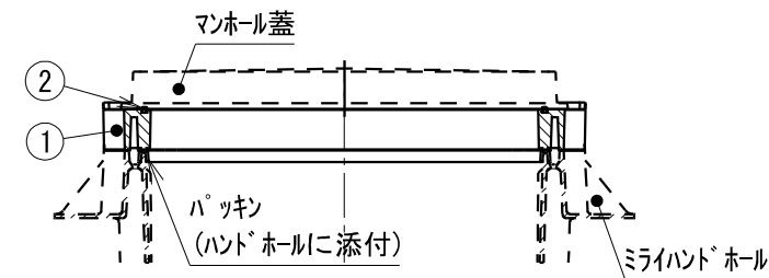
施工状態参考図
