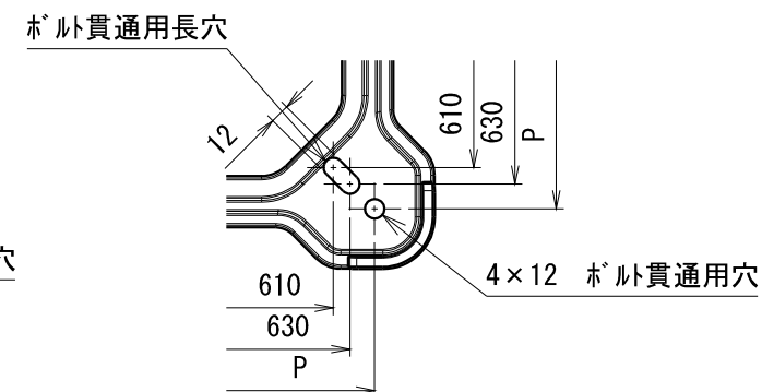
MH-600-50 ボルト貫通部詳細
